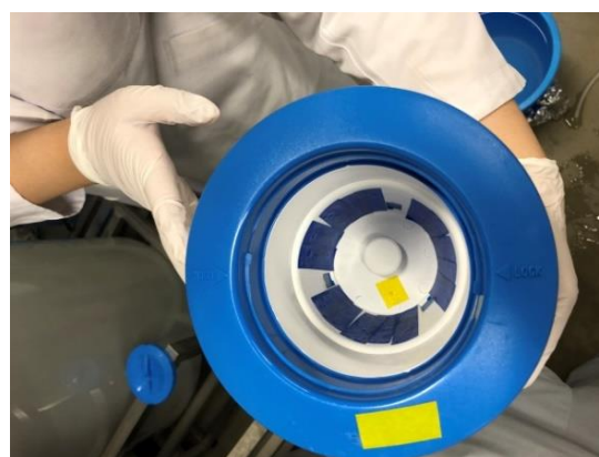
写真 4 塩素溶解速度の調整例（内部）
